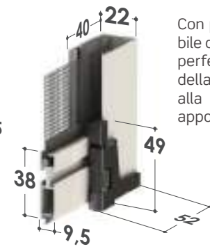
Cassonetto da 42
