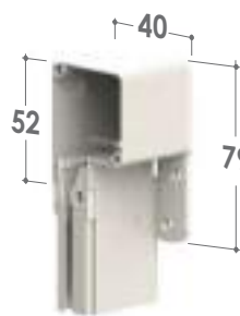
Cassonetto da 40
