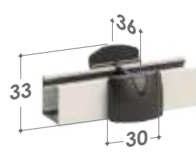
VERSIONE DOPPIA
