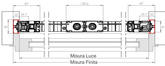
Apertura bilaterale
