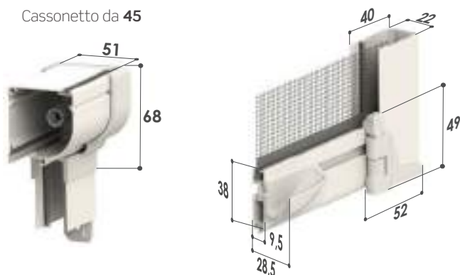
Cassonetto da 45
