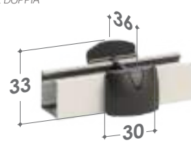
VERSIONE DOPPIA
