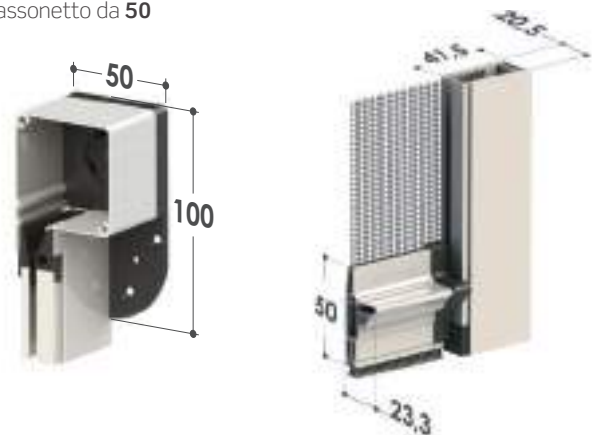
Cassonetto da 50
