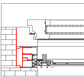
SEZIONE ORIZZONTALE
