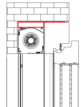
SEZIONE VERTICALE
