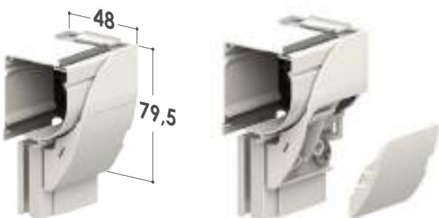
Cassonetto da 45
