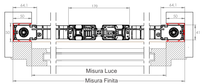
Chiusura centrale
