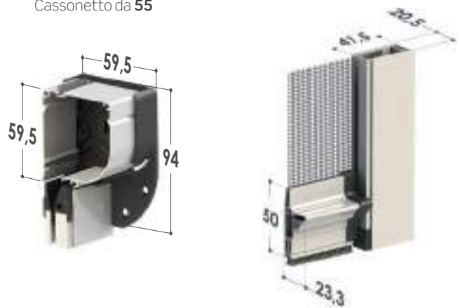
Cassonetto da 55
