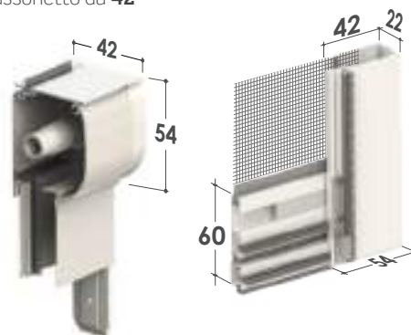
Cassonetto da 42
