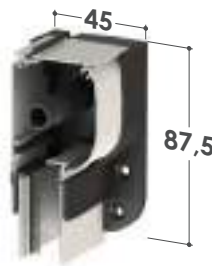
Cassonetto da 42
