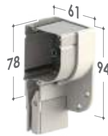
Cassonetto da 55
