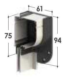
Cassonetto da 55
