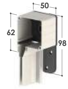
Cassonetto da 50
