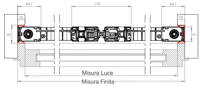
Chiusura centrale
