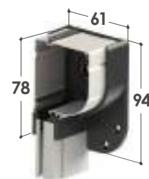
Cassonetto da 55
