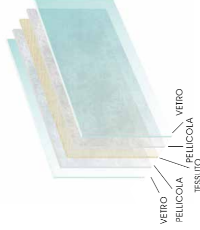
Vetro stratificato con tessuto fra 2 vetri.
