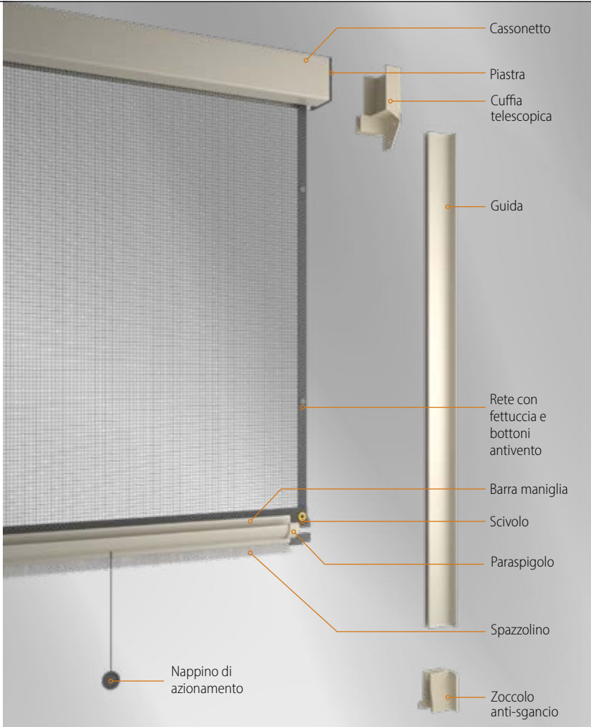
Cuffie telescopiche
