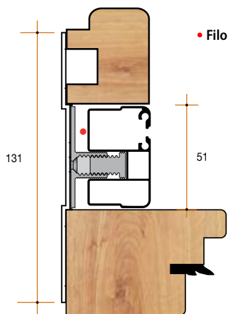
Esempio con guida e compensatore basso
