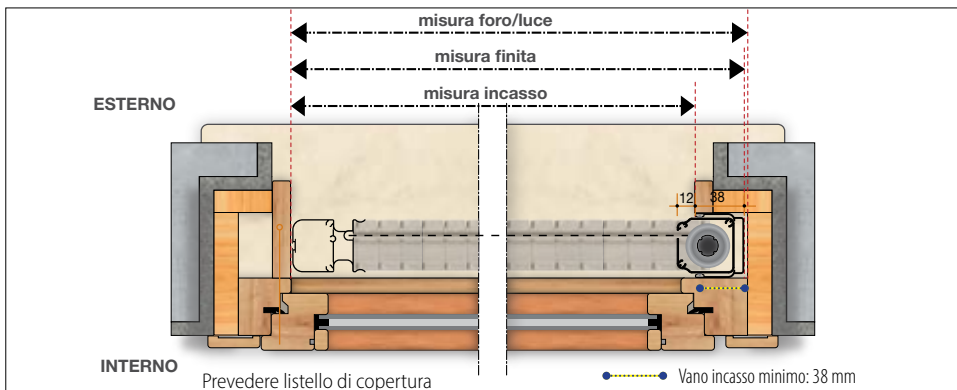
Sezione orizzontale con opzione "Incasto 2 lati".
