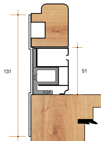
Esempio con guida e compensatore modello Delta
