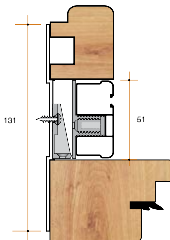
Esempio con guida e compensatore alto
