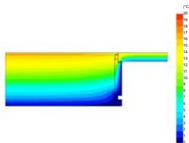
Slim Restauro - Spalla
