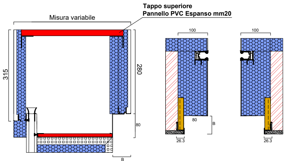
CASSONETTO IE con Spalla a filo cassonetto ringrossata
