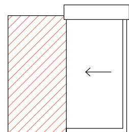
UNISLIDE : Telaio a scomparsa laterale a 1 anta e Monoblocco con Cassonetto e Guide
