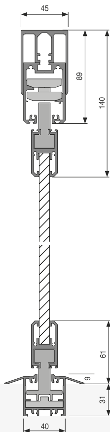
Sezione verticale guida incassata
