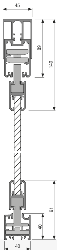
Sezione verticale guida superficie
